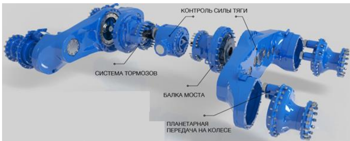
Рис.5 Сочлененные(балансирные) мосты фирмы NAF
