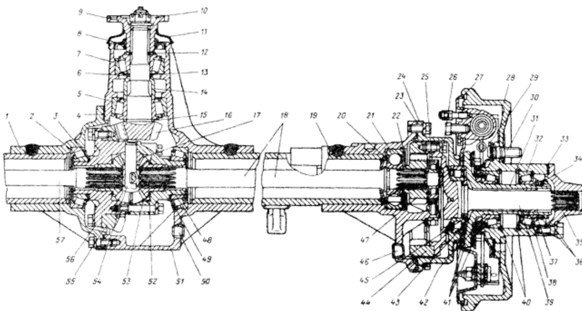
Рис. 4. Задний мост автомобиля УАЗ-3151
