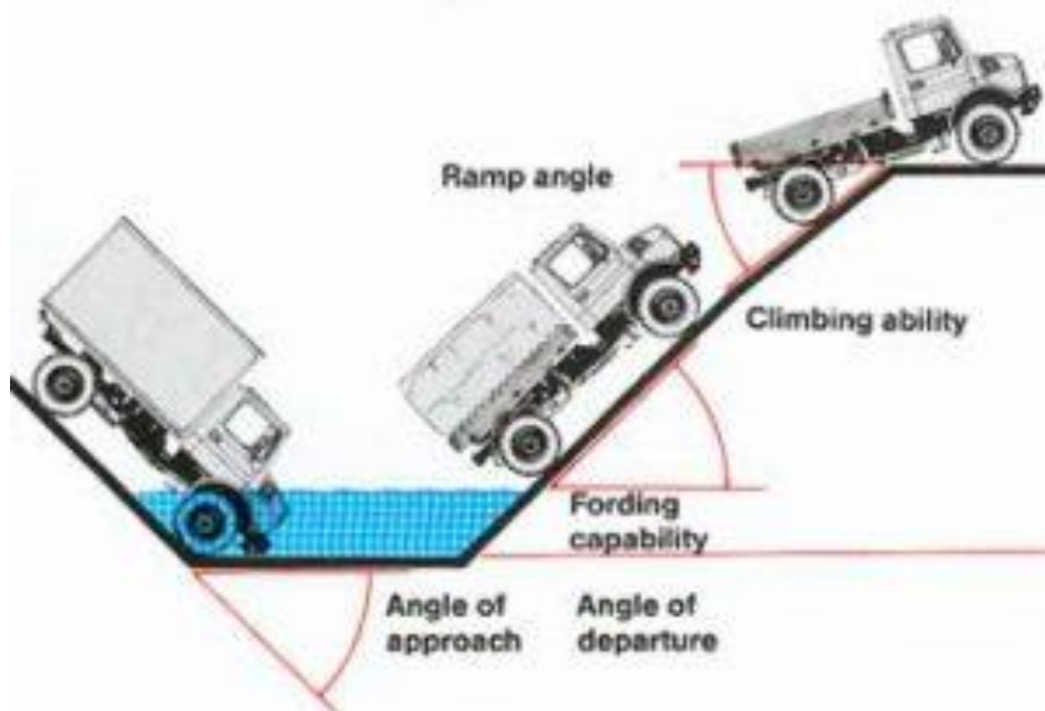
Рис.2. Углы въезда, съезда и рамп современного автомобиля Unimog.
