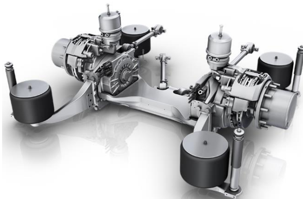
Рис.7. U-образных мост для автобуса фирмы ZF
