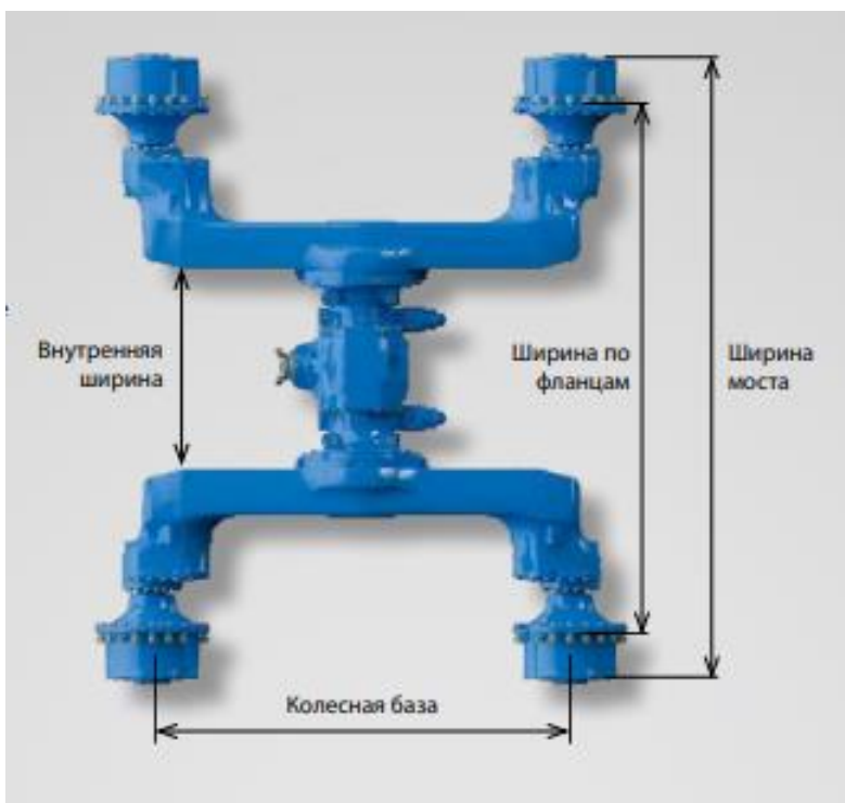
Рис.6. Мост NAF в сборе
