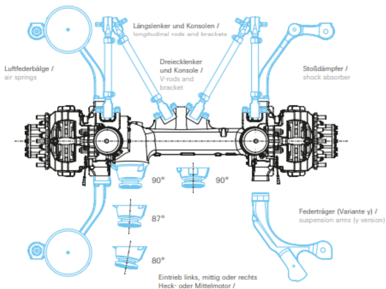
Рис.8. Общий вид моста ZF с электроприводом
