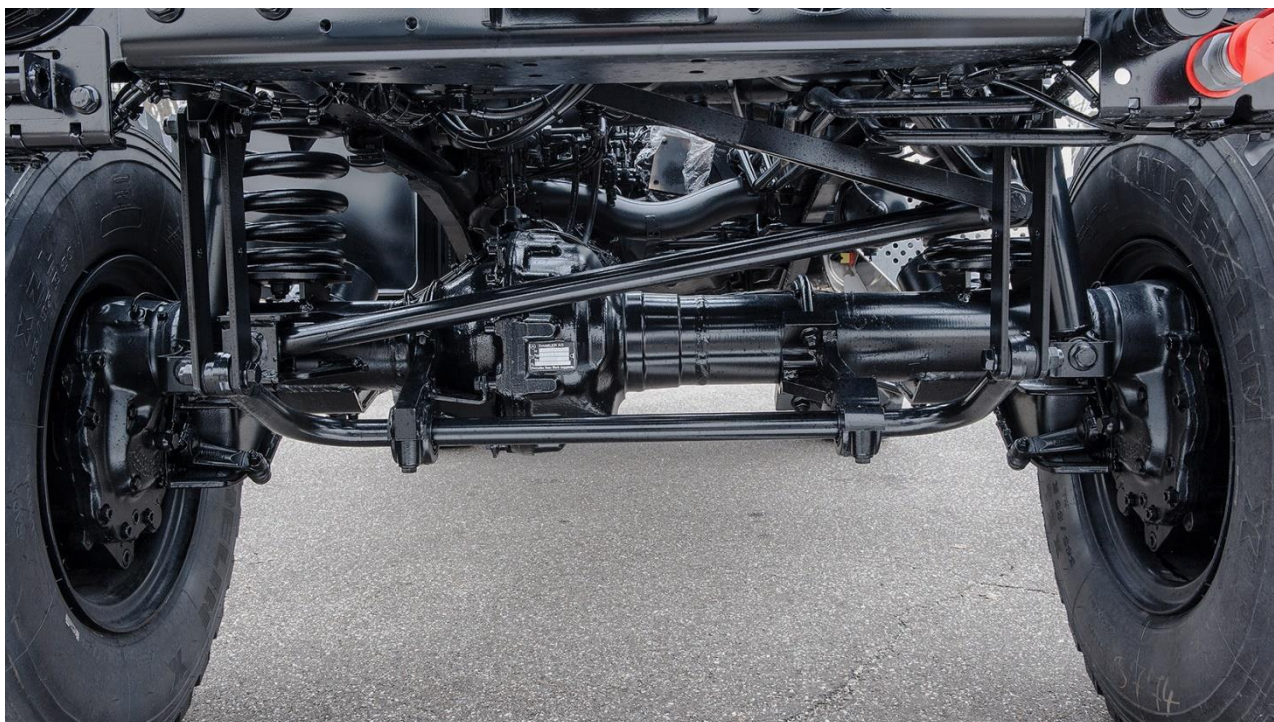
Рис.3 Ведущий мост автомобиля Mercedes-Benz Unimog U 500
